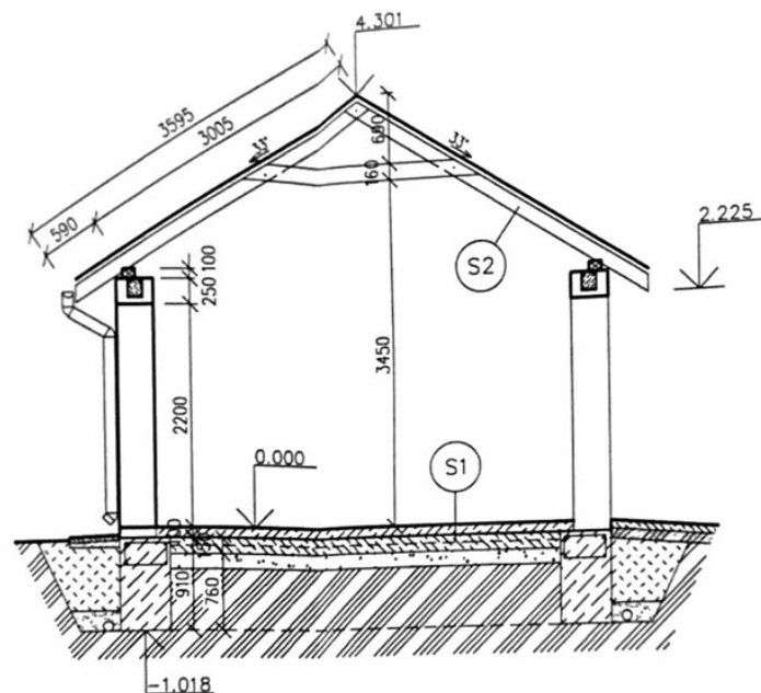
ŘEZ A-A
